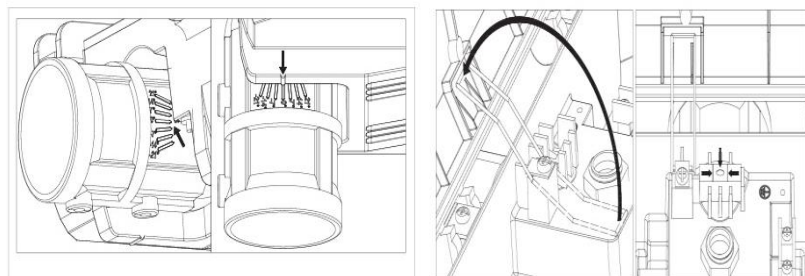
Horizontaler Einbau
